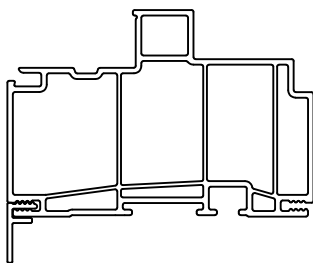
1/2" FLUSH FIN
