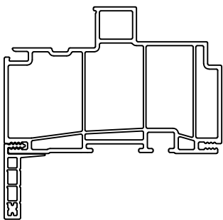
1" FLUSH FIN
